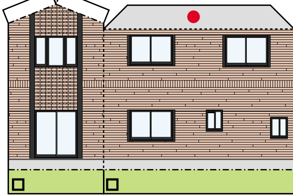
南側壁
