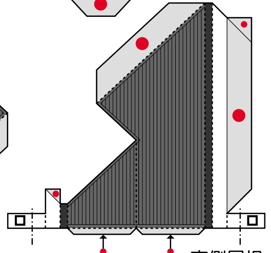
東側屋根
