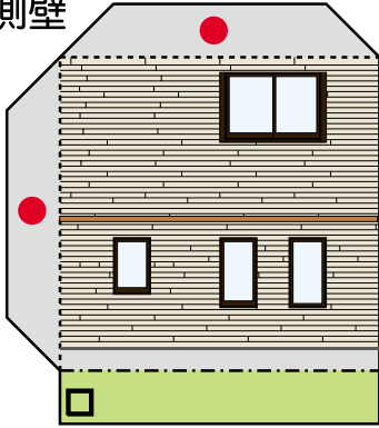
北側壁
